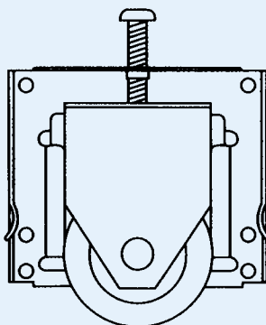
WVG300 DOOR ROLLER
